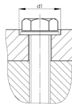
DIN 974 T2 Reihe 3 (DIN 74 Form R)
